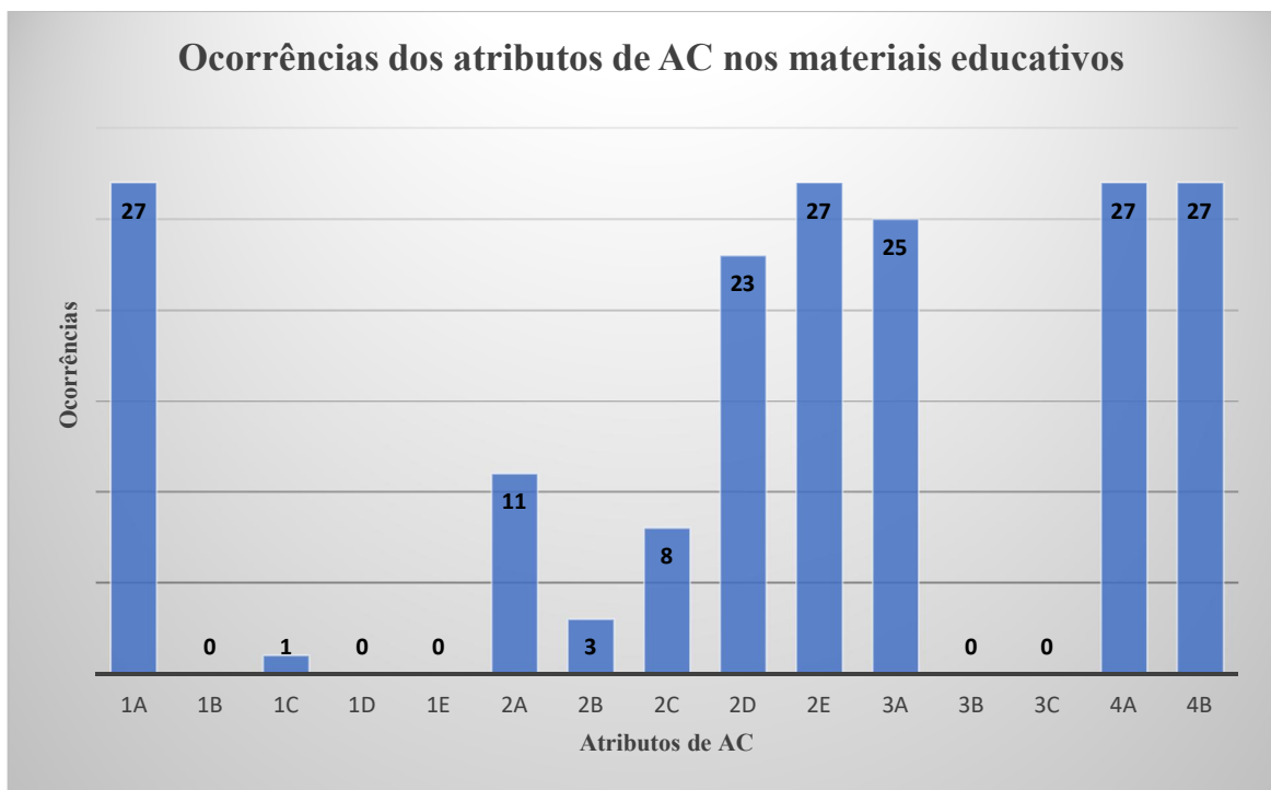
Figura 30: Gráfico da ocorrência dos atributos de AC nos materiais educativos do Zôo de Sorocaba
